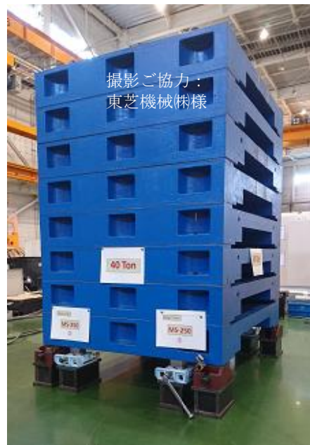
荷重 40 トンを支え実施のデモ
