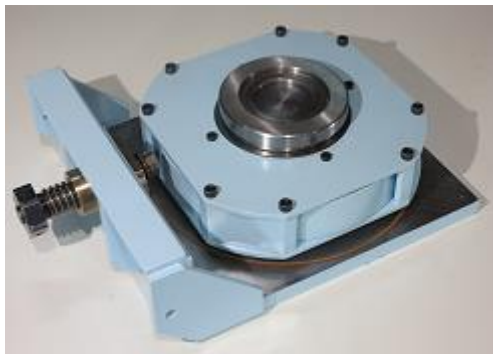
マジカル・スライド MS-25T (側面送りジャッキ付)
